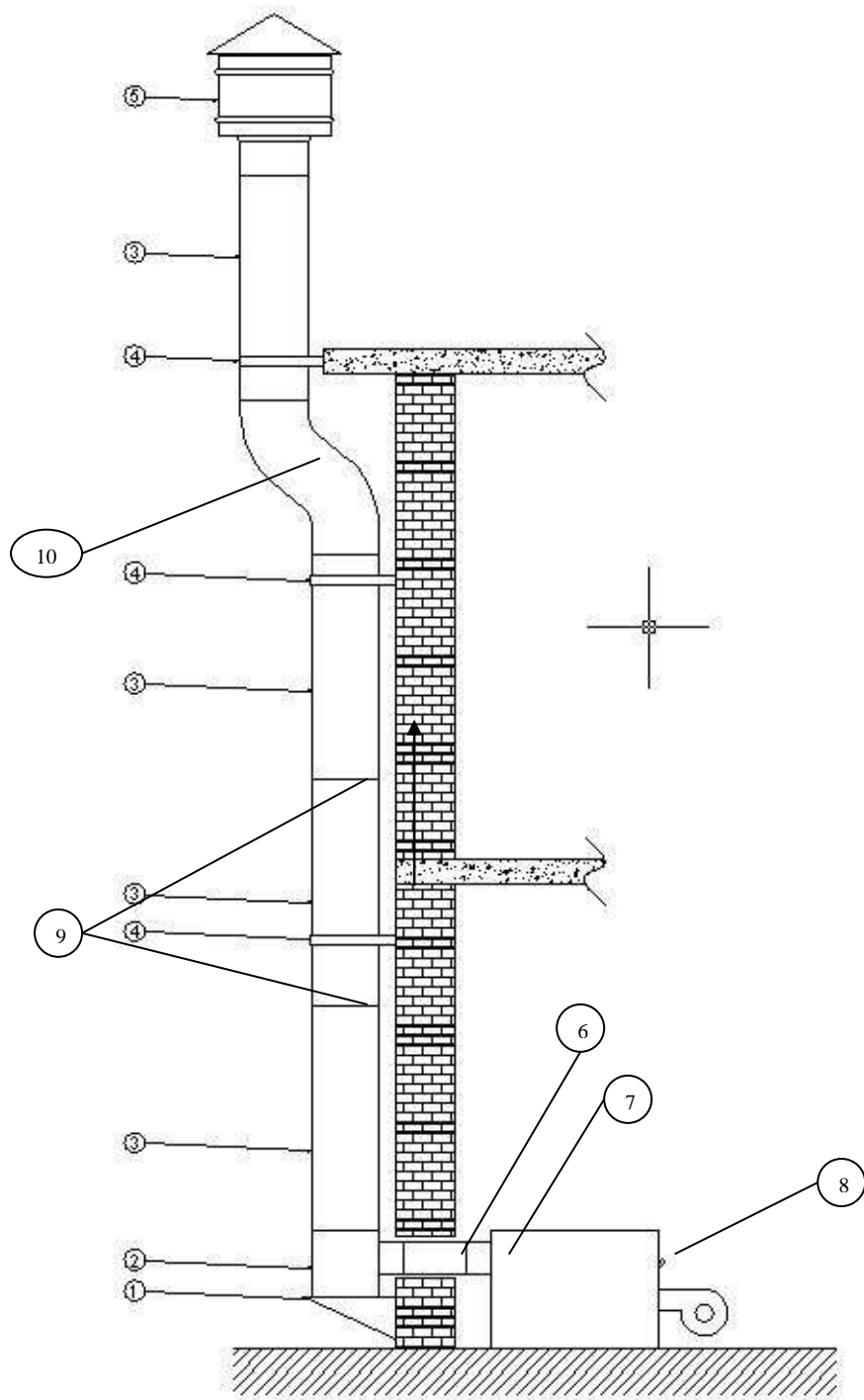
Εικόνα 1. Τυπική εγκατάσταση (εξωτερικής) καμινάδας
